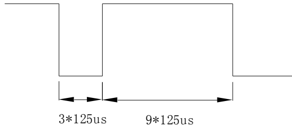
图 2-1 面板向主板发送“0”的定义
