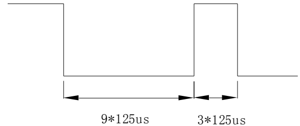
图 2-2 面板向主板发送“1”的定义
