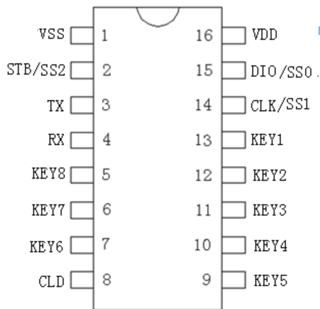
图 5-1 GRM807FNS_02 管脚图
