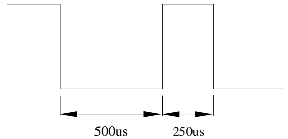
图 3-2 主板向面板发送“1”的定义
