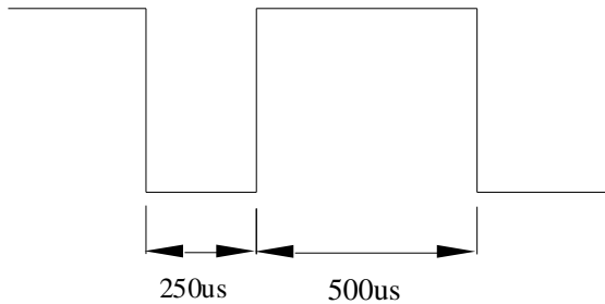
图 3-1 主板向面板发送“0”的定义
