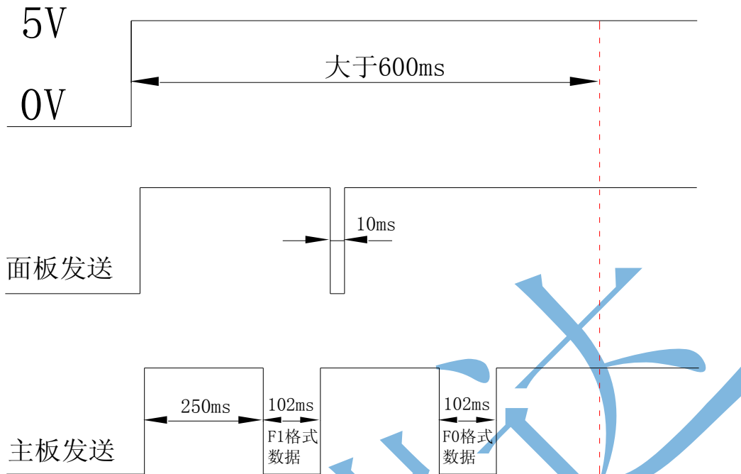
图 5-1 逻辑时序
